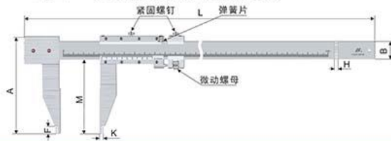
矩形管尺身圆弧爪游标卡尺0-2000mm
