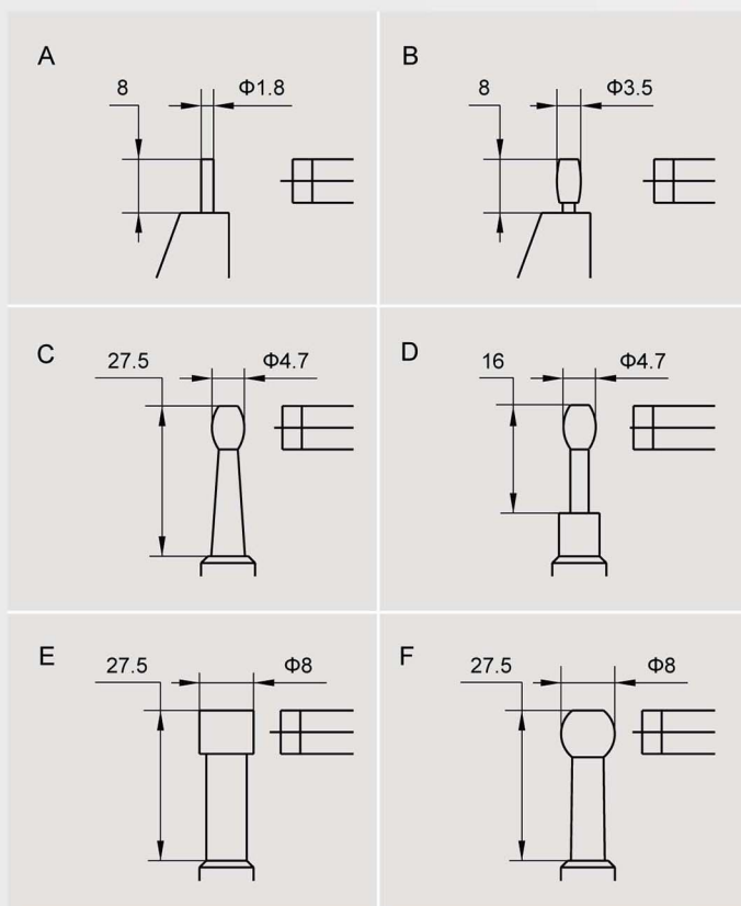
测量壁厚
